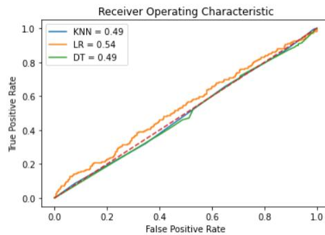
Fig. 3 ROC- AUC curve
