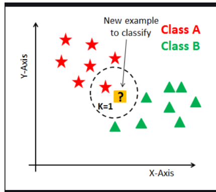
Fig.1 - KNN
