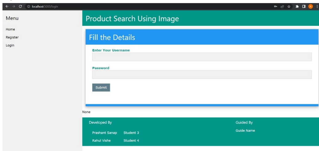
Fig. 2: Login Page
