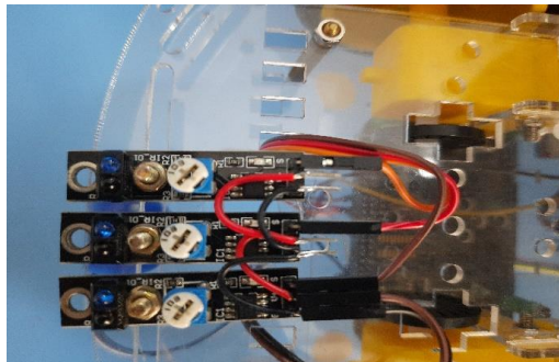
Fig. 1. IR sensor
